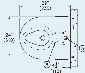
2125A-T-3-FM SIPHON JET
